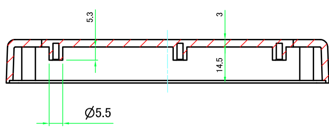
F-F ( 1 : 1.5 )
